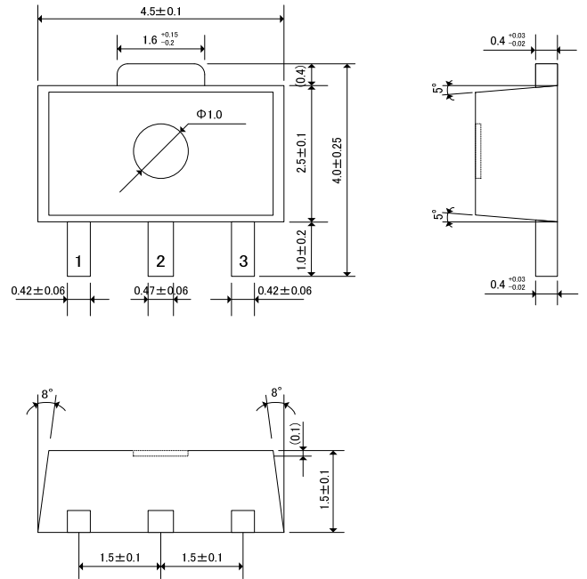
SOT-89
